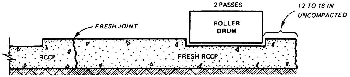
(1) ROLL 1 FT FROM EDGE
